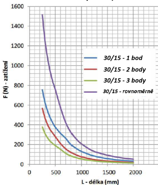
NOSNÍK 30/15 x 1,25 mm
